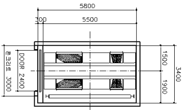
출입구 평면도
