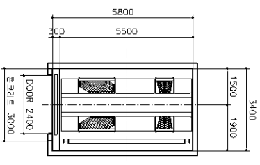
종인구 평면도
