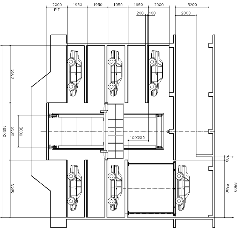
측면도
