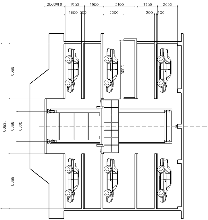
측면도
