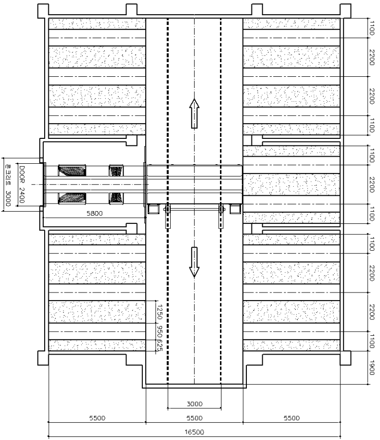
평면도
