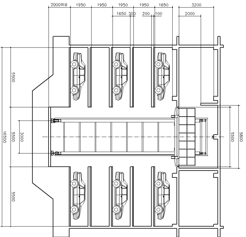
측면도
