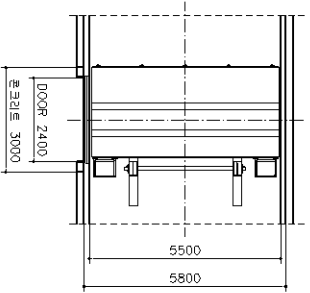
출입구 평면도
