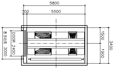
트럭용 평면도
