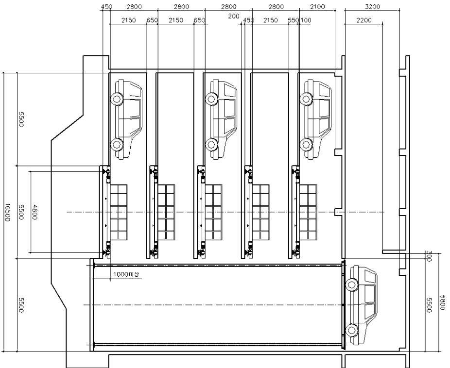
측면도
