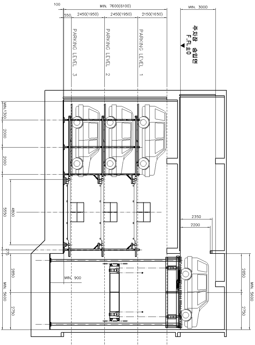
주차장 측면도
