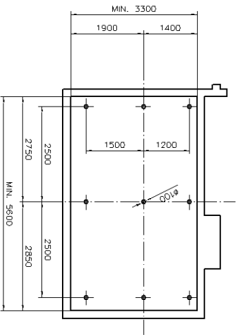
설치용 CABIN 천정 HOLE 위치도
