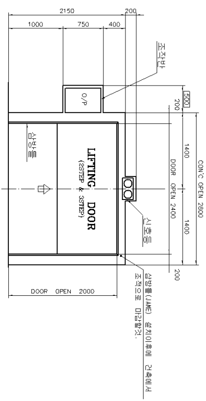
출입구 골조 시공도
