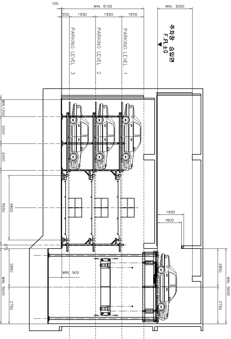
주차장 축면도
