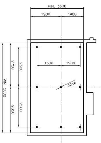
설치용 CABIN 천정 HOLE 위치도
