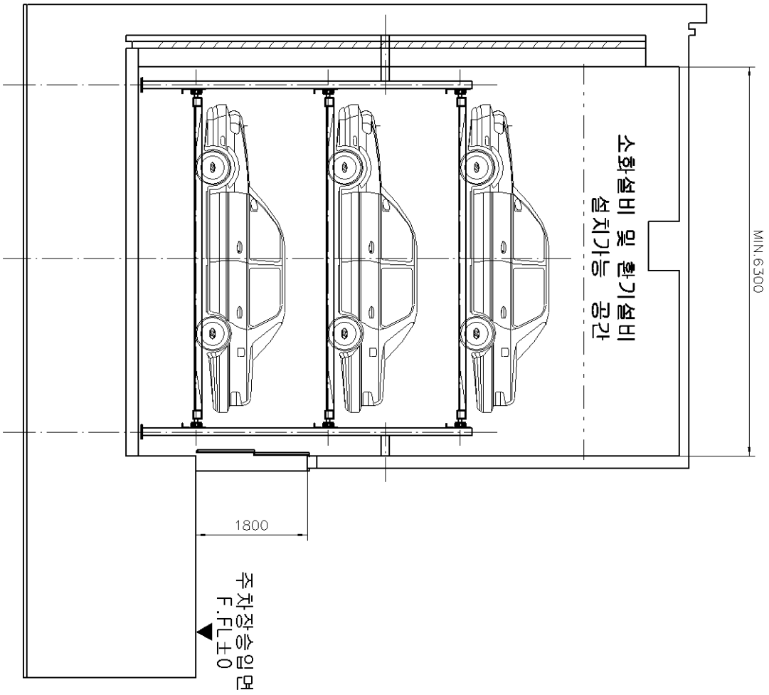
주차장 측면도
