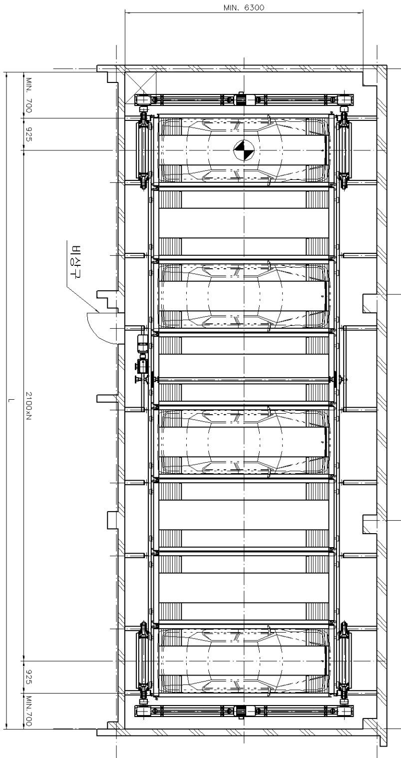
주차층 평면도
