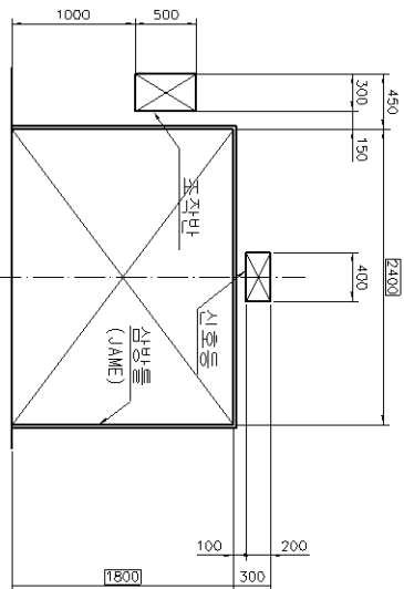
입고층 개구부 상세도
