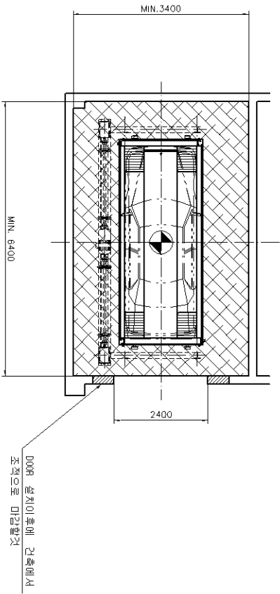
주차장 입고층 평면도
