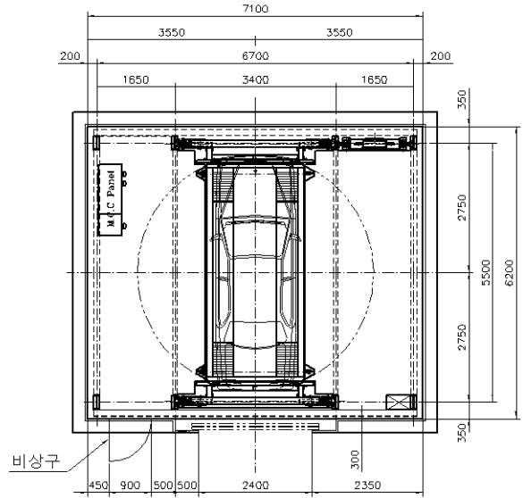
입고층 평면도
