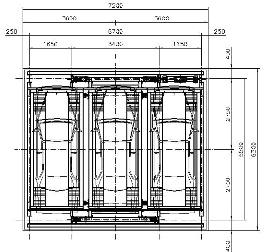
기준층 평면도
