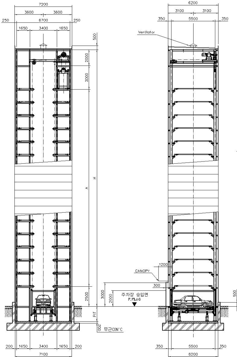
주차장 정면도
