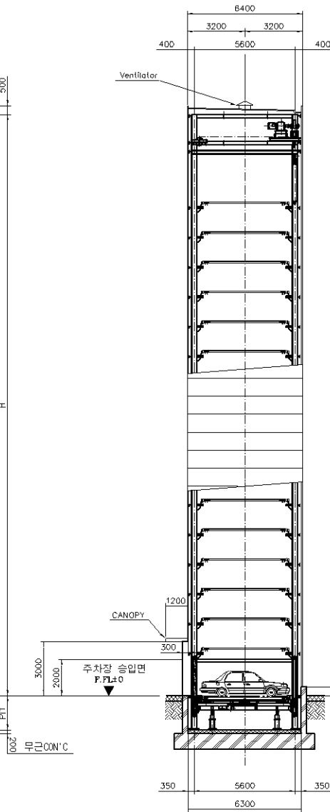
주차장 측면도
