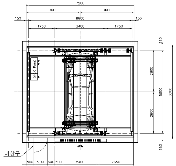
입고층 평면도
