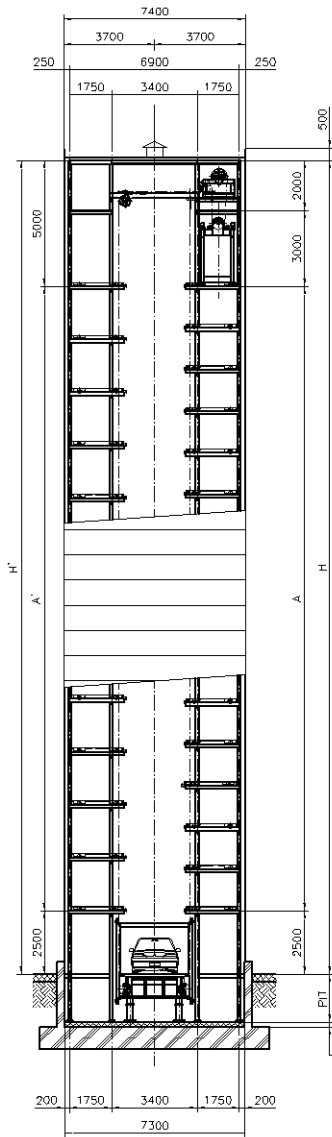
주차장 정면도
