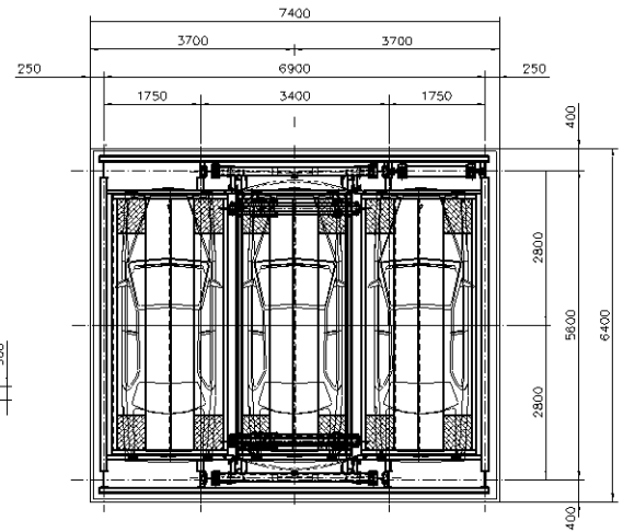
기준층 평면도
