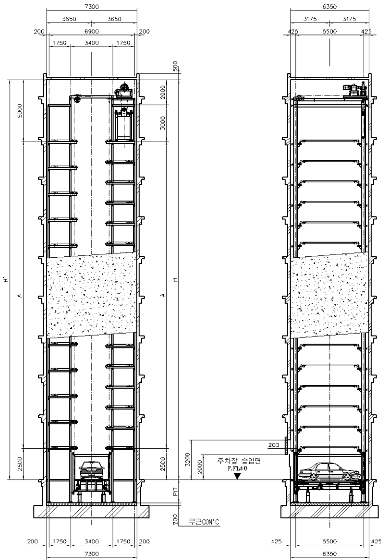
주차장 정면도
