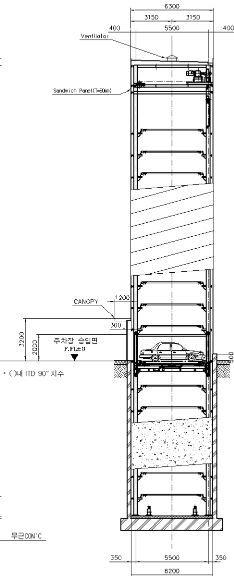
주차장 측면도
