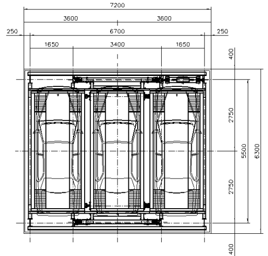
기준층 평면도
