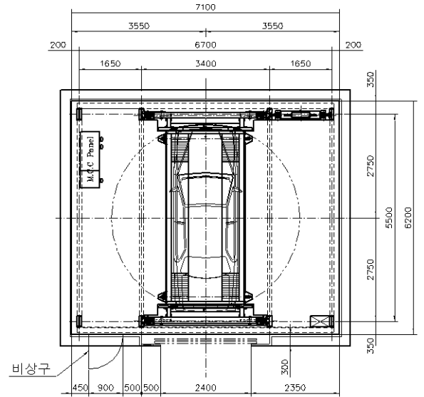
입고층 평면도
