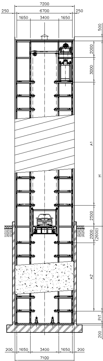
주차장 정면도
