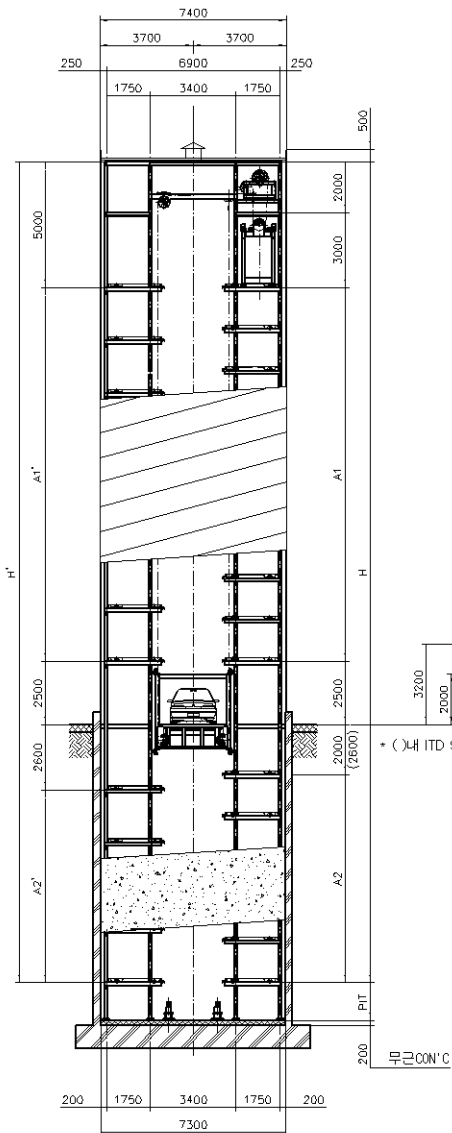
주차장 정면도
