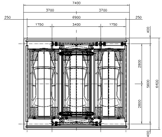
기준층 평면도
