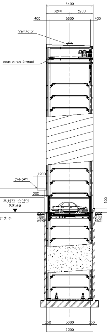
주차장 측면도
