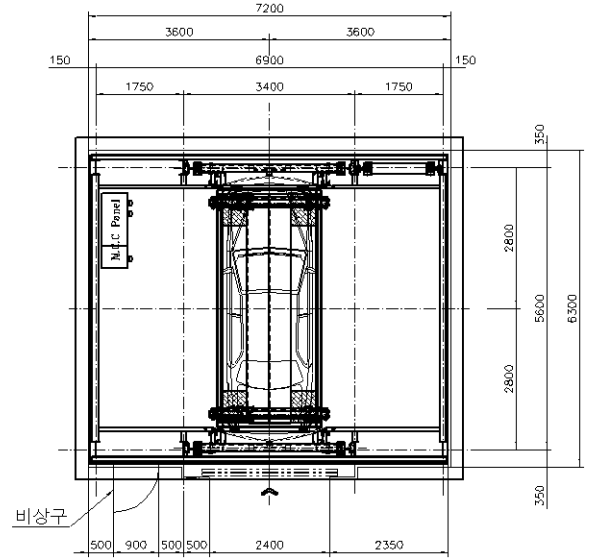
입고층 평면도
