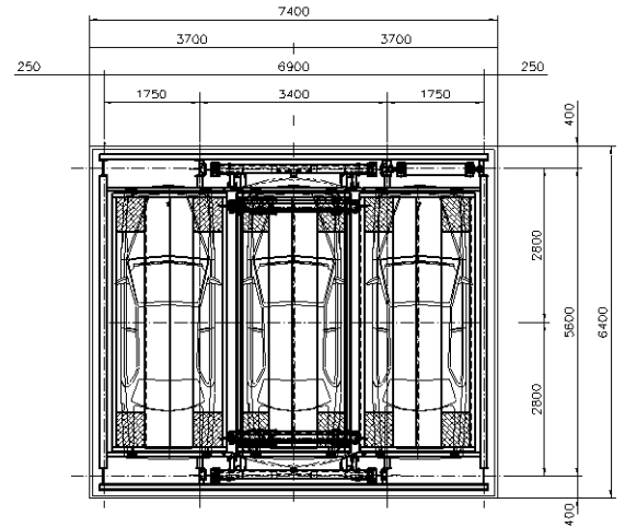
기준층 평면도
