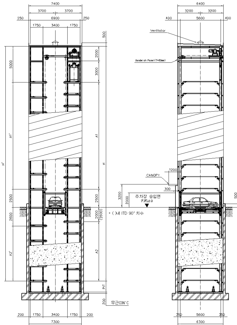
주차장 정면도
